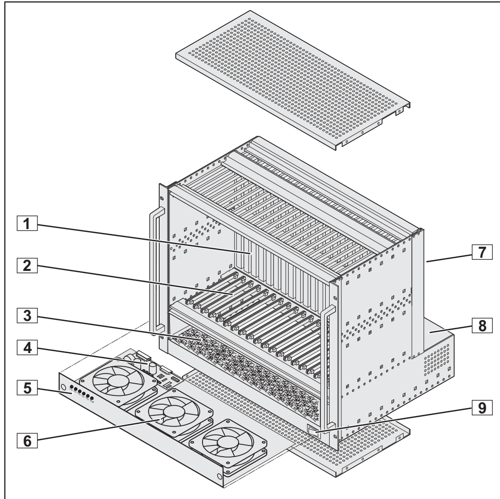
Figure 1: Ansicht vorn
