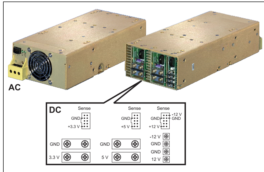
Figure 2: Netzteil
